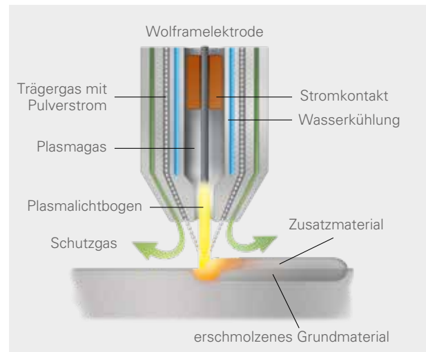
Direct Energy Deposition - Arc (DED-Arc) mit Pulver
