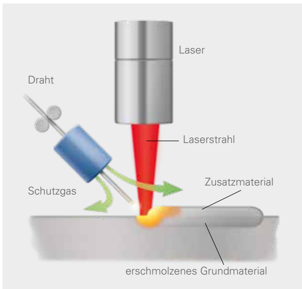
Direct Energy Deposition - Laser Beam (DED-LB) mit Draht
