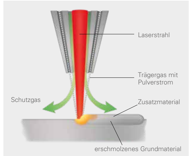
Direct Energy Deposition - Laser Beam (DED-LB) mit Pulver
