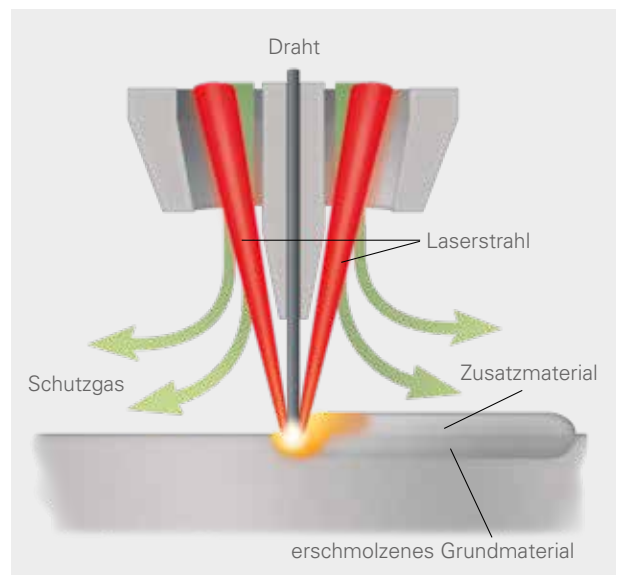
Koaxiales Direct Energy Deposition - Laser Beam (DED-LB) mit Draht
